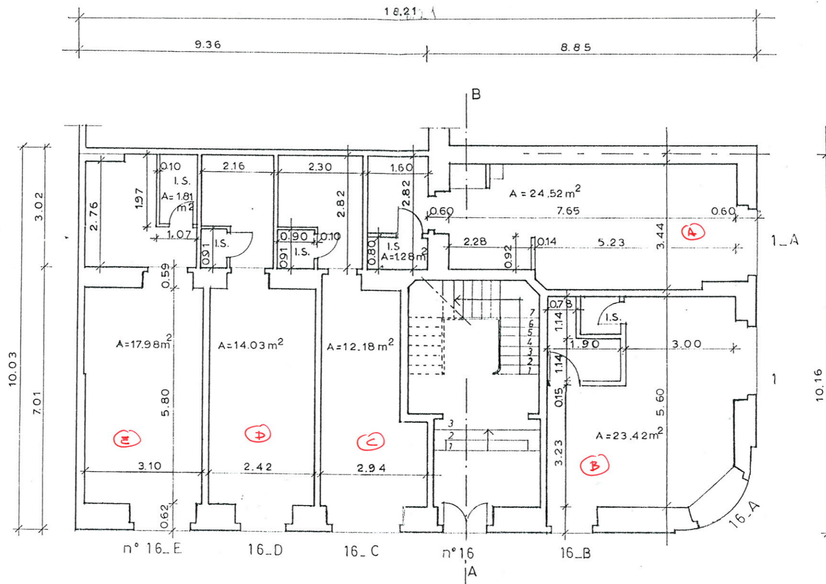
PLANTA DAS LOJAS — R/C
